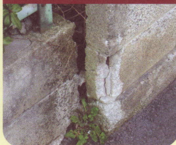
笠木の壊れや土圧
